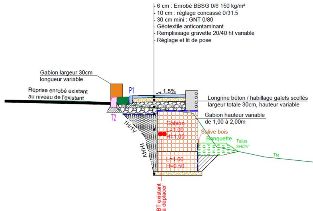
- Vue en Coupe du mur à créer
