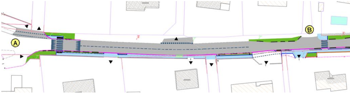
- Vue en plan de l'impasse des Burlats au Sq Lesdigières
