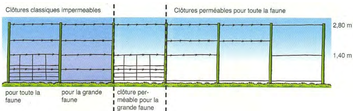
Schéma de différents types de clôtures perméables à la faune. Illustration : G. Crisci.
